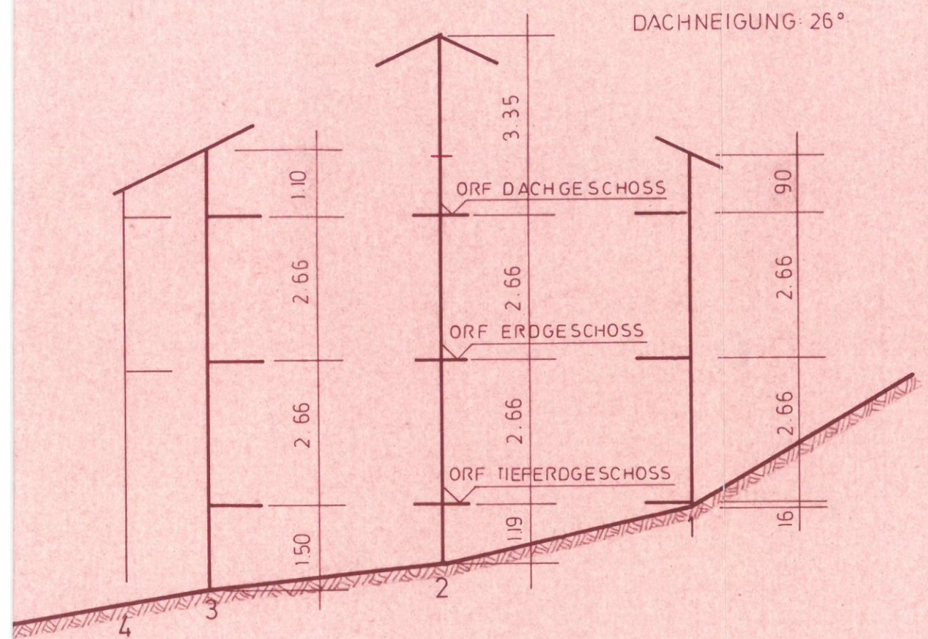
OSTGIEBEL IM M 1:100
